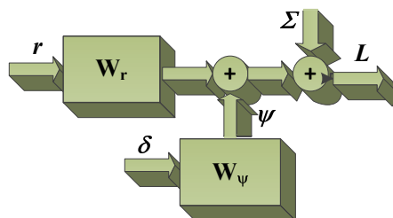
Рисунок 4 – Структурна схема лінійної моделі підсистеми inv\_cp
