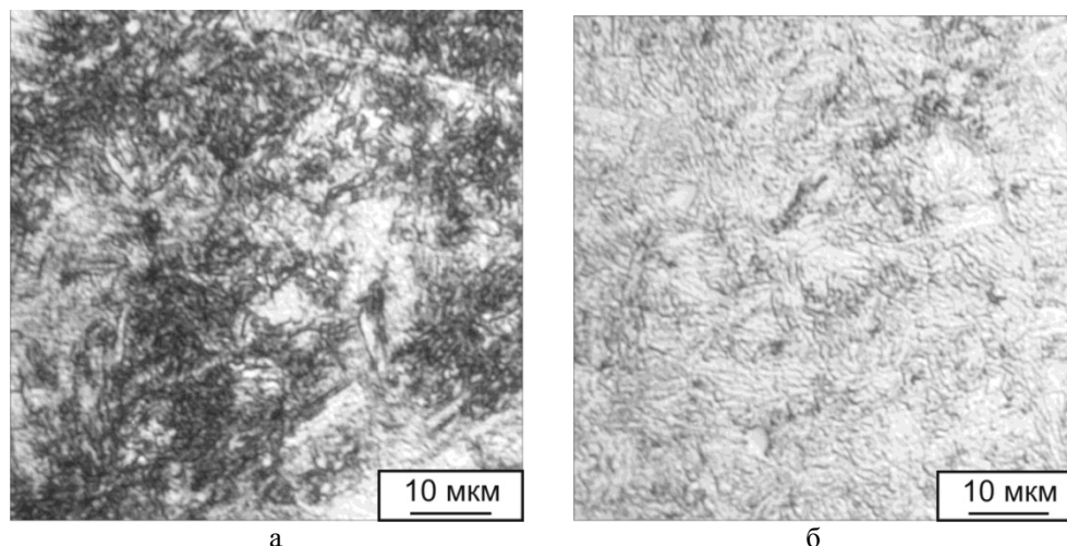
Рисунок 4 – Мікроструктура сталі після термічної обробки:
