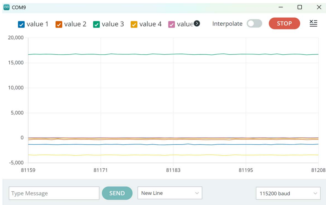
Рисунок 2 – Експериментальні сигнали у часі сирих інерціальних даних, зчитаних з двох MEMS-модулів MPU-6500 у режимі механічного спокою макетного стенда
