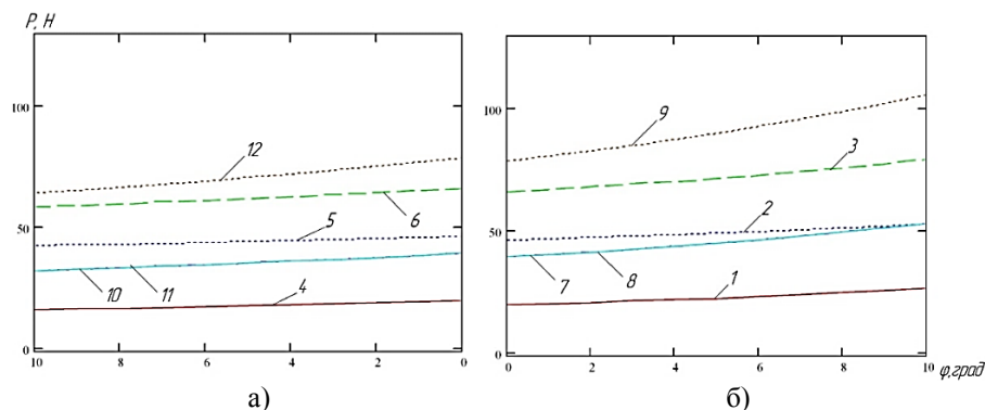
а) - вершина призми зміщена в сторону від захватного пристрою; б) - вершина призми зміщена в сторону захватного пристрою.
