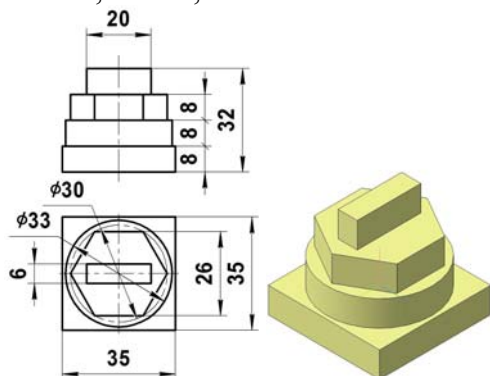
Рисунок 2 – Зразок з охоплюваними валами характерної форми
