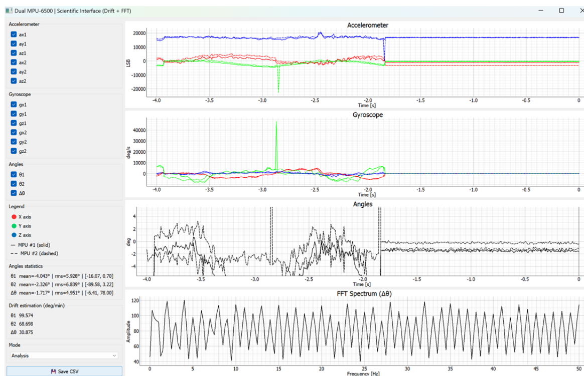
Рисунок 5 – Остання модернізація GUI для реєстрації та обробки експериментальних досліджень Джерело: розроблено авторами
