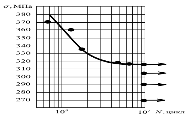
Рисунок 6 - Крива втоми сплаву ВТ1-0 після обробки азотуванням (група №3)
