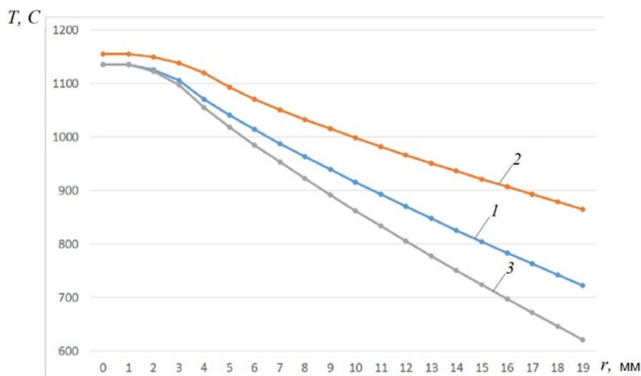
Рисунок 2 – Розподіл температури у виливку кулі Ø40 мм при повному затвердінні (чавун виробу: 2,5 % C, 1 % Si; товщина стінки сферичної моделі чавунного кокіля – 40 мм) 1 – базовий варіант моделювання (шар фарби 0,5 мм з розрахунком газового зазору); 2 – варіант порівняння (товщина облицювання 1 мм з розрахунком газового зазору); 3 – нефарбований кокіль (без розрахунку газового зазору). Джерело: розроблено авторами
