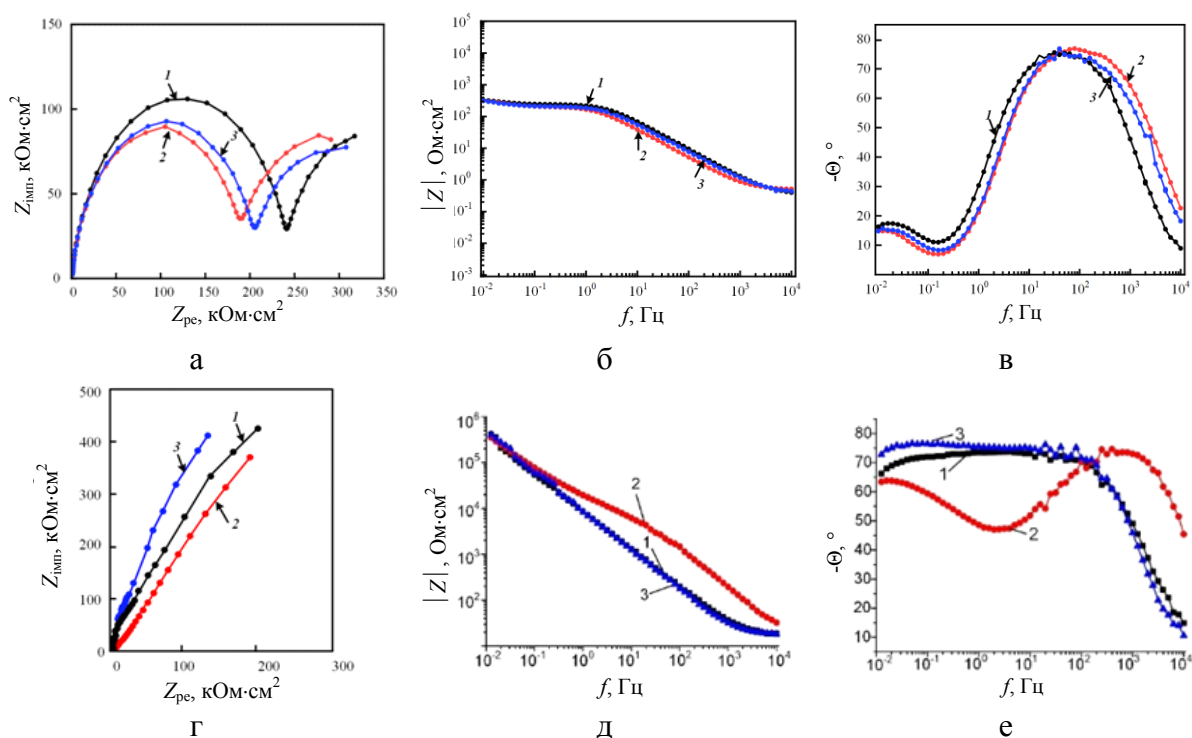
а, г – Графіки Найквіста; б, в, д, е – Бode; а-в – 20%-ий розчин хлоридної кислоти; г-е – розчин Рінгера; 1 – традиційно у вихідному стані; 2 – 3D друком у вихідному стані; 3 – 3D друком після термічної обробки
