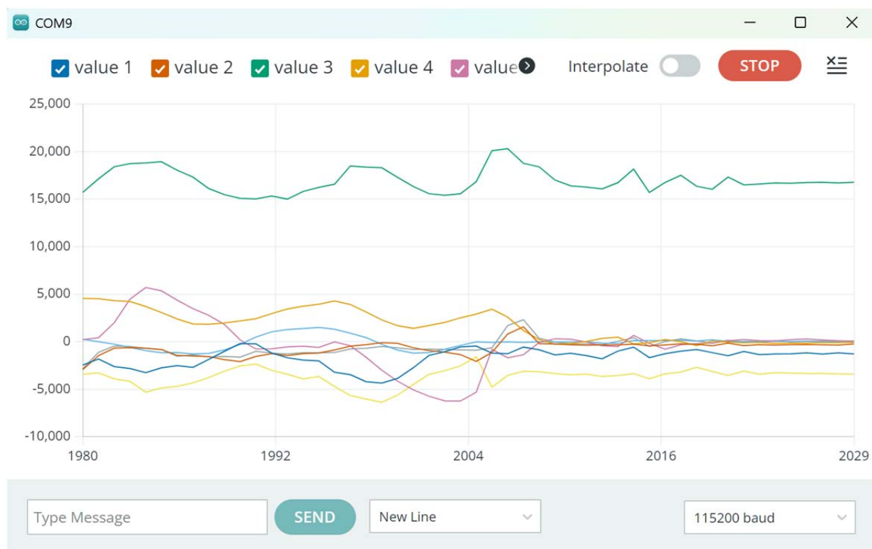
Рисунок 3 – Експериментальні сигнали сирих інерціальних даних при прикладенні зовнішнього механічного впливу до макетного стенда
