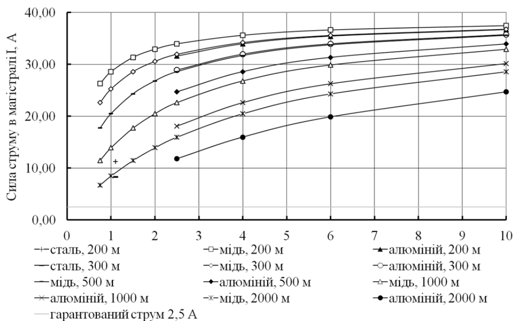
Рисунок 2 – Залежність сили струму в магістральному провіднику електропровідної мережі від його параметрів за змінної напруги 380 В
