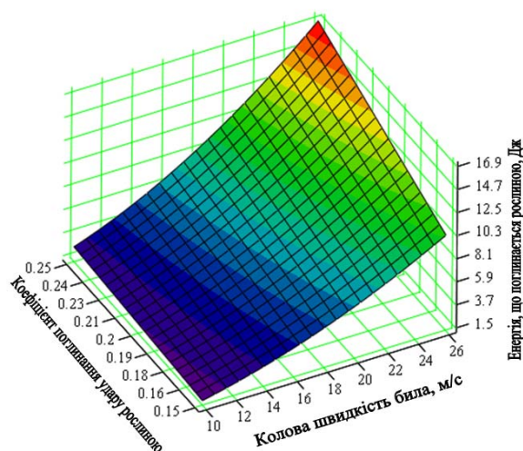
Рисунок 1 – Графічна залежність поглинання енергії рослиною при дії била Джерело: розроблено авторами
