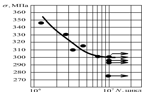
Рисунок 7 - Крива втоми сплаву ВТ1-0 після обробки
