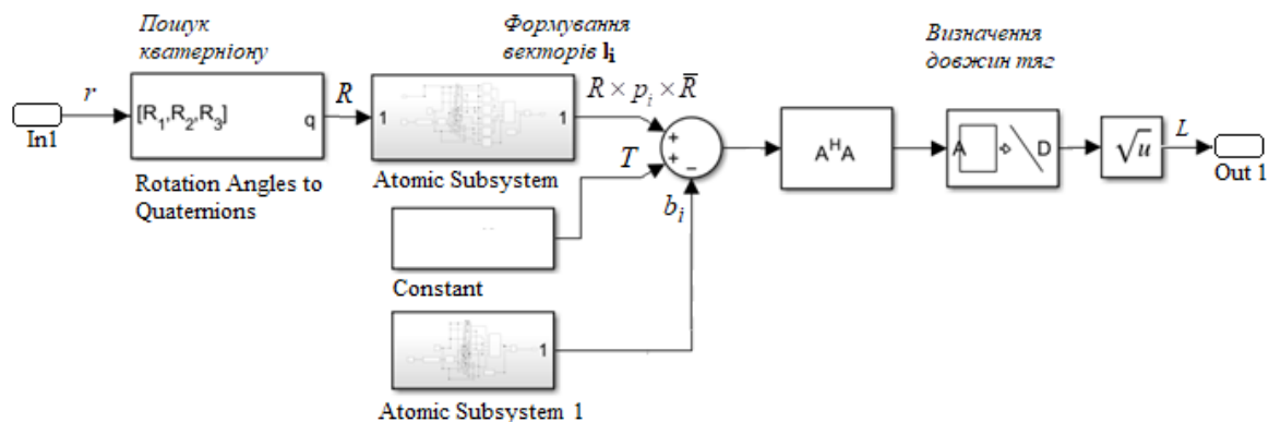
Рисунок 3 - Підсистема розв'язання зворотного завдання кінематики
