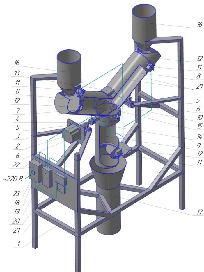
1 – станина; 2 – кроковий двигун; 3 – гнучка муфта; 4 – вал; 5 – корпусні підшипники на лапах; 6 – гумові демпфери; 7 – Y-подібна ємність; 8 – нахилені патрубки; 9 – прямий патрубок; 10 – фітинг-трійник; 11 – сервоприводи; 12 – заслінки; 13 – акселерометр; 14 – струмопровідне контактне кільце; 15 – розподільник; 16 – завантажувальні патрубки; 17 – вивантажувальний патрубок; 18 – блок живлення; 19 – контролер крокового двигуна; 20 – блок керування з дисплеєм; 21 – клавіатура; 22 – електричні проводи; 23 – кнопка вмикання
