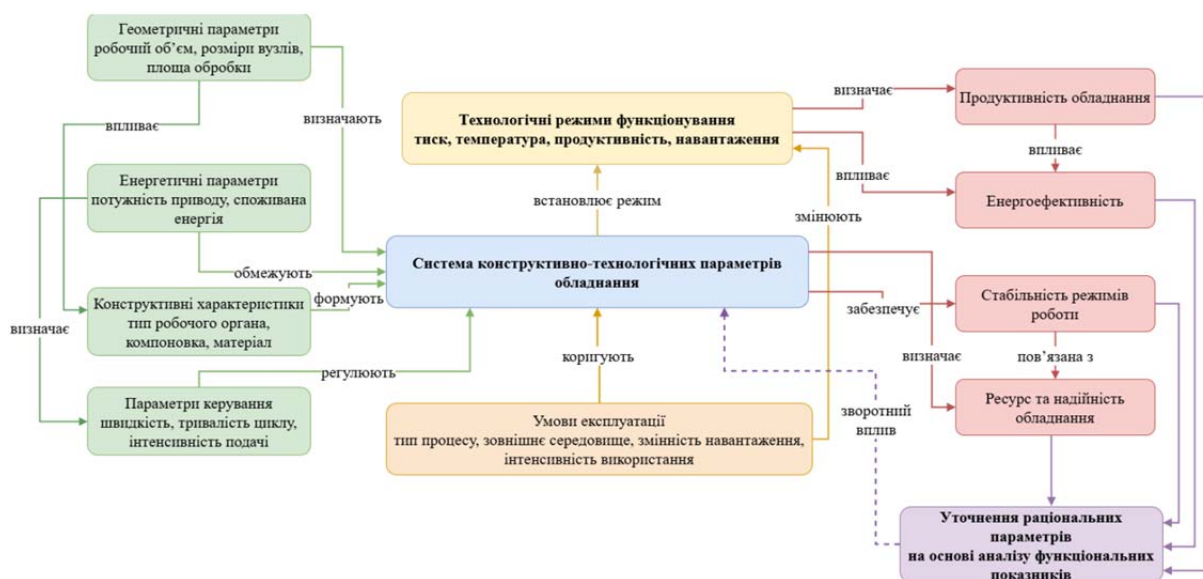
Рисунок 2 – Взаємозв'язок конструктивно-технологічних параметрів обладнання аграрного виробництва
