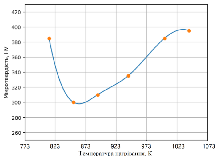
Рисунок 5 – Зміна твердості сталі після ізотермічної витримки в бейнітній області (723 К) та подальшим нагріванням в інтервалі 803...1053 К.
