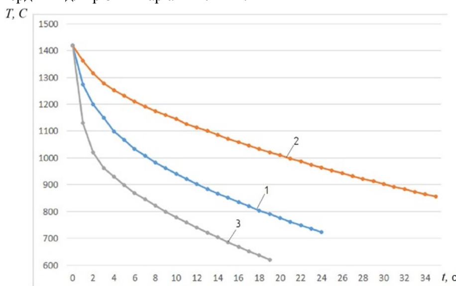
Рисунок 3 – Розрахункова зміна температури поверхневого шару виливка чавунної кулі Ø40 мм до повного затвердіння (чавун виробу: 2,5 % C, 1 % Si; товщина стінки сферичної моделі чавунного кокіля – 40 мм)
