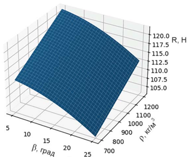
Рисунок 6 – Залежність тягового опору лапи від кута атаки \beta і щільності ґрунту \rho
