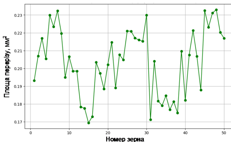
Рисунок 1 – Графік середньої площі перерізу зерна від його номера
