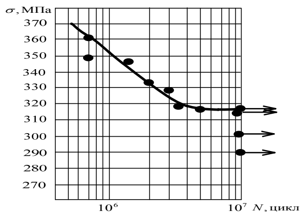
Рисунок 8 - Крива втоми сплаву ВТ1-0 після обробки азотуванням (група №5)
