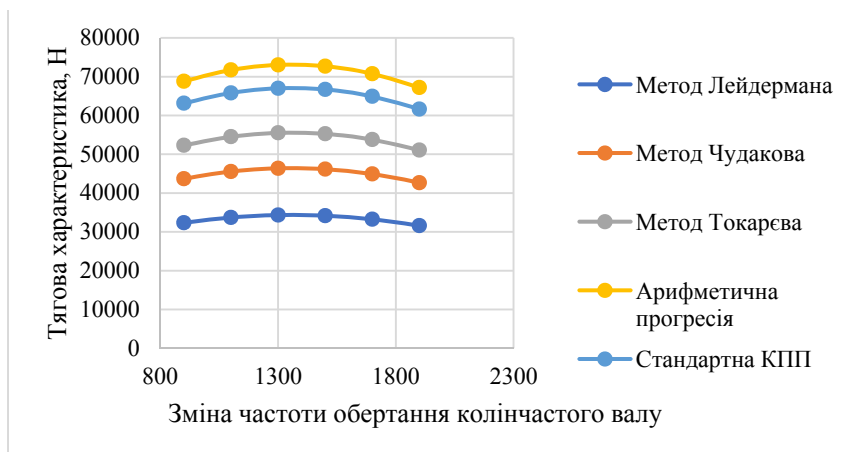
Рисунок 3 – Тягові характеристики автобуса на четвертій передачі при використанні різних методик формування передавального ряду коробки передач Джерело: розроблено автором
