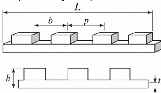
Рисунок 1 – Конструкція дослідної пластини та контрольовані геометричні параметри Джерело: розроблено автором
