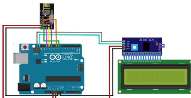
Рисунок 5 – Схема під'єднання дисплея 1602 до модуля nRF24L01 ARDUINO
