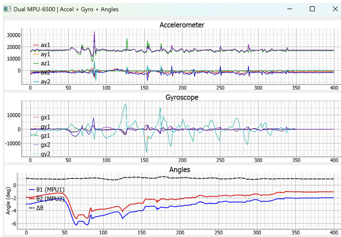
Рисунок 4 – Модернізація GUI №3, додавання графіка Angle до графічного інтерфейсу
