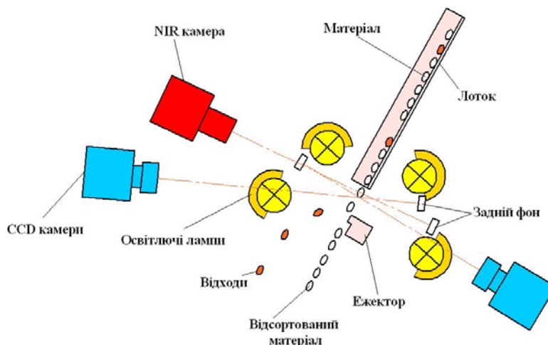
Рисунок 2 – Технологічна схема роботи фотосепаратора
