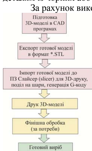
Рисунок 1 – Порядок створення готової деталі
