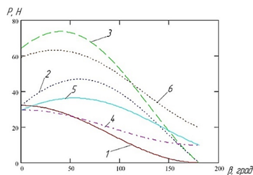
Рисунок 3 – Графіки впливу напрямку сили інерції (β) на сили затиску (P)
