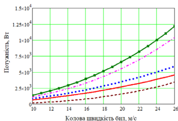
Рисунок 2 – Криві складових потужностей, що витрачаються на привод ротаційного барабана Джерело: розроблено авторами
