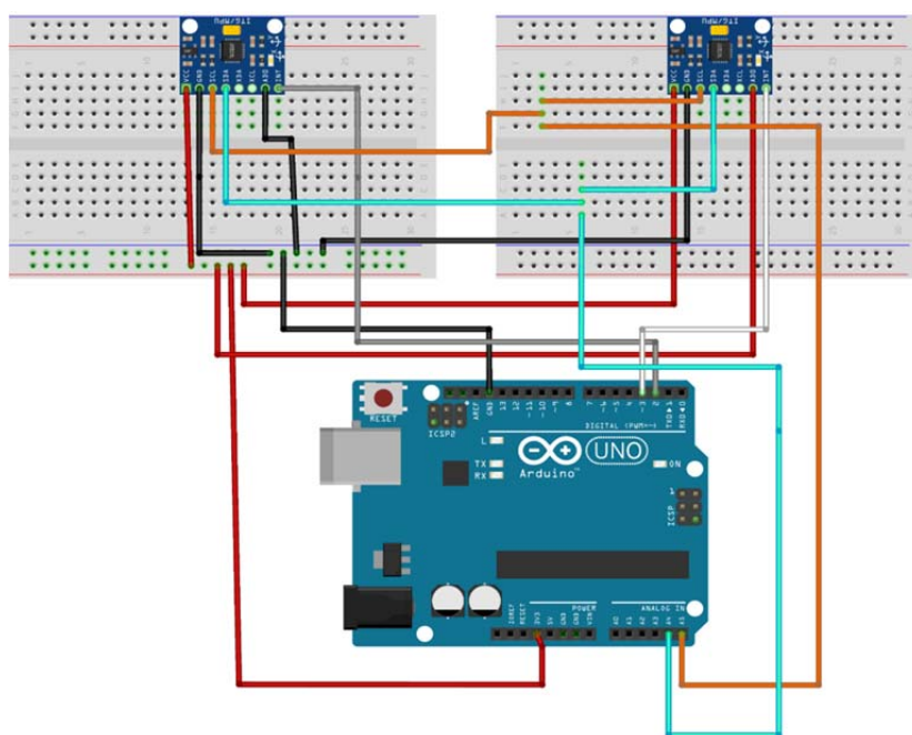
Рисунок 1 – Макетний стенд збору інерціальних даних на основі плати Arduino Uno та двох MEMS-модулів MPU-6500, підключених спільною шиною I 2 C
