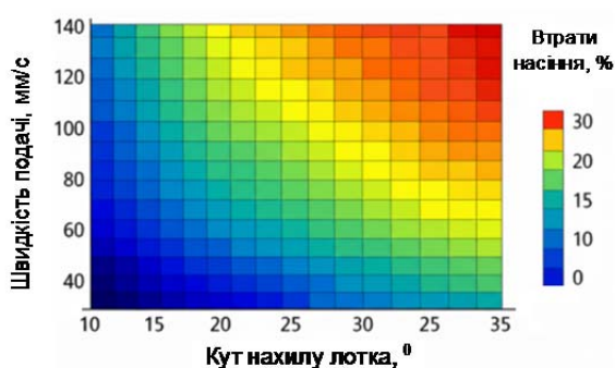
Рисунок 7 – Вплив кута нахилу лотка та швидкості подачі на втрати насіння ріпаку
