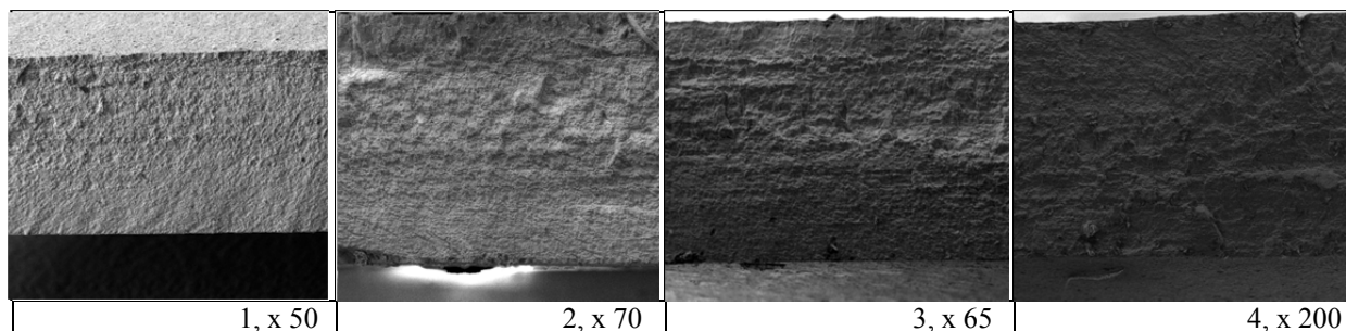
Рисунок 2 - Злом від втоми титанового сплаву ВТ1-0 після модифікації методом вакуумного іонного азотування в імпульсному режимі: – при T = 390^\circ\text{C} ; 2 – при T = 473^\circ\text{C} ; 3 – при T = 590^\circ\text{C} ; 4 – при T = 750^\circ\text{C} .
