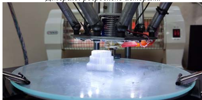
Рисунок 6 – Друк дослідних зразків на 3D-принтері DELTA-FDM
