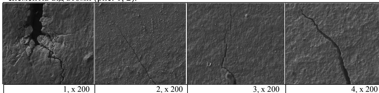
Рисунок 1 - Розвиток тріщини по поверхні зразка з Ті-сплаву: при температурі 750°C: 1 – до азотації (ВТ1-0); 2 – після азотації (ВТ1-00); 3 – до азотації (ВТ1-00); 4 – після азотації (ВТ1-00).
